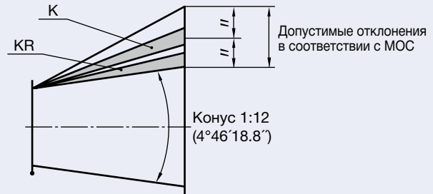
Рис. 7.2 Допустимые отклонения
