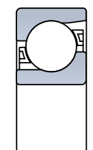
Поперечное сечение подшипника TAC03AT85
