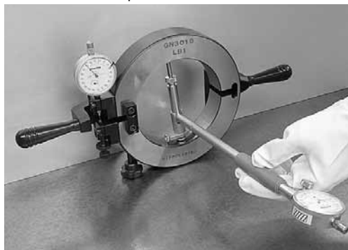
Рис. 1.11 Регулировка вписанного диаметра калибра GN
