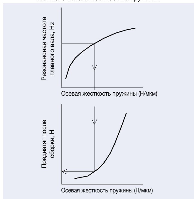
Рис. 1.28 Взаимосвязь между резонансной частотой главного вала и жесткостью пружины
