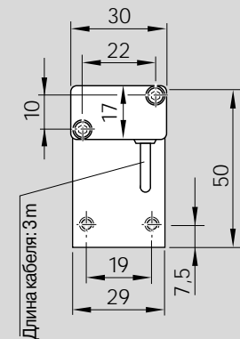
Индуктивный выключатель с монтажной арматурой для рамы размером -110
