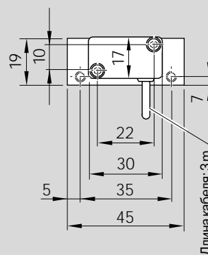
Индуктивный выключатель с монтажной арматурой для рамы размером -65, -80, -165
