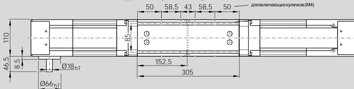
Длинная каретка с Т-образными пазами
