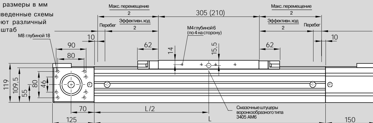
Длинная каретка с Т-образными пазами
