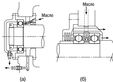
Рис. 12.8. Смазка впрыскиванием
