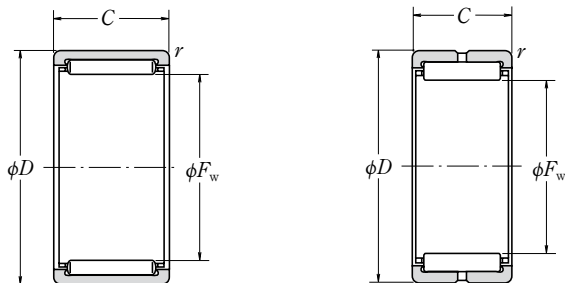
RLM Без внутреннего кольца
