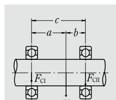
Подшипник I Подшипник II Рисунок 5.5. Распределение радиальной нагрузки (1)
