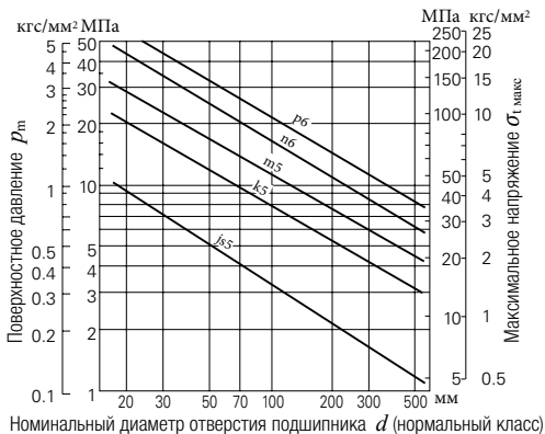
Рис.15.5. Поверхностное давление p_m , а также максимальное напряжение \sigma_{T \text{ макс}} для среднего натяга
