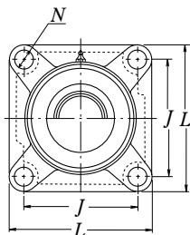
Тип со стальной штампованной пьезозащитной крышкой
