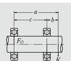
Подшипник I Подшипник II Рисунок 5.6. Распределение радиальной нагрузки (2)
