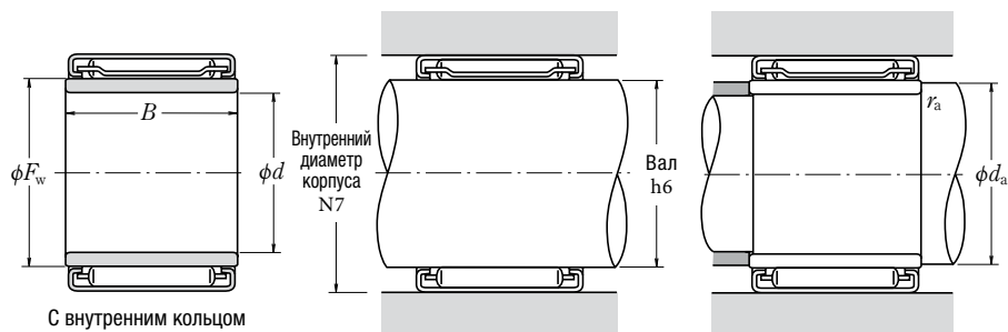
С внутренним кольцом
