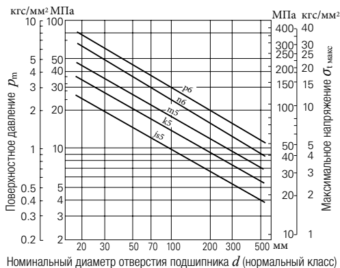
Рис.15.6. Поверхностное давление p_m , а также максимальное напряжение \sigma_{T \text{ макс}} для максимального натяга
