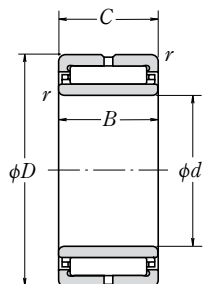
С внутренним кольцом NA
