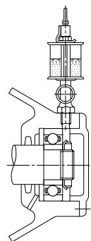
Рис. 12.5. Капельное смазывание
