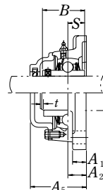
Тип с литой пьезозащитной крышкой
